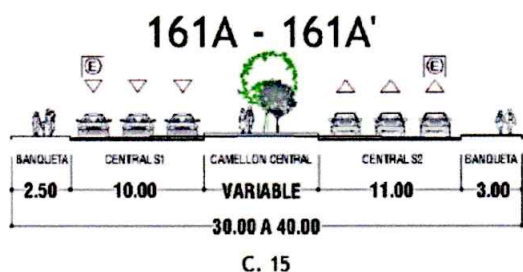
Figura 22. Sección Vial Calle 15ª. PDU 2040 Sexta Actualización.
