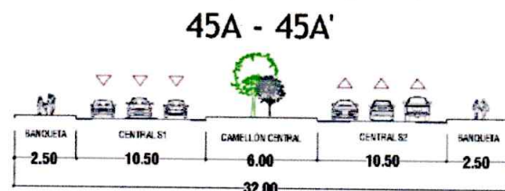
Figura 36. Sección vial Boulevard José Fuentes Mares. PDU 2040 Sexta Actualización.
