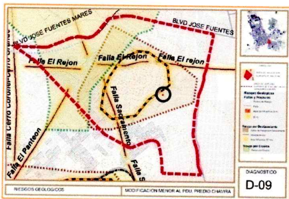
Figura 32. Fallas geológicas. Con respecto a área de estudio P.D.U. 2040 Sexta Actualización.
