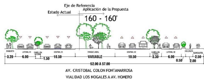
Ilustración 38. Av. Tecnológico también conocida como Av. Cristobal Colón Fontarrosa y su sección actual. Fuente: PDU 2040 y Google Earth, 2022.
