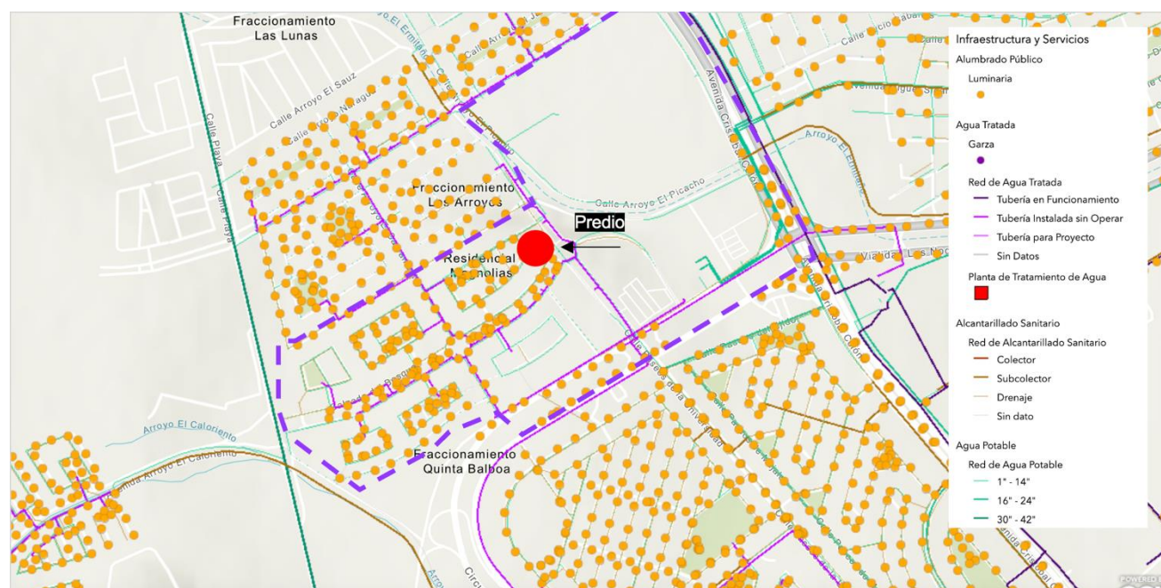
Ilustración 42. Plano de infraestructura existente. Fuente: SIGMUN, 2022.
