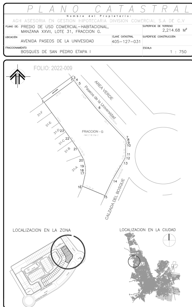
Ilustración 8. Plano Catastral y cuadro de construcción.
