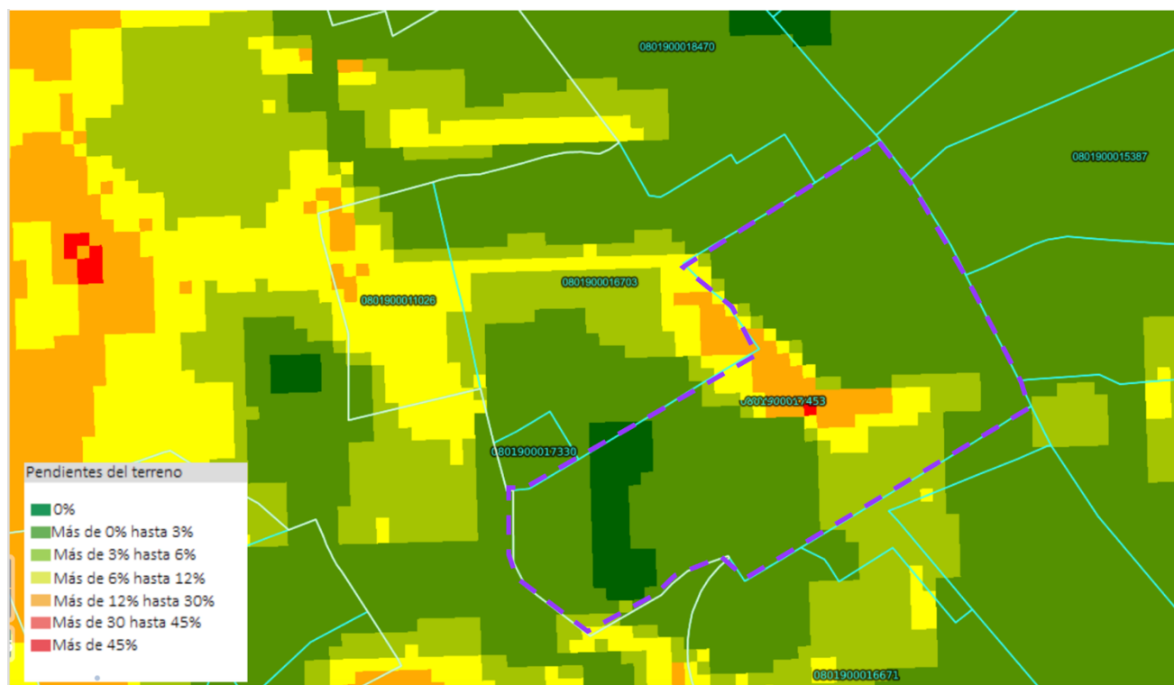
Ilustración 22. Topografía y pendientes de terreno. Fuente: PDU 2040.
