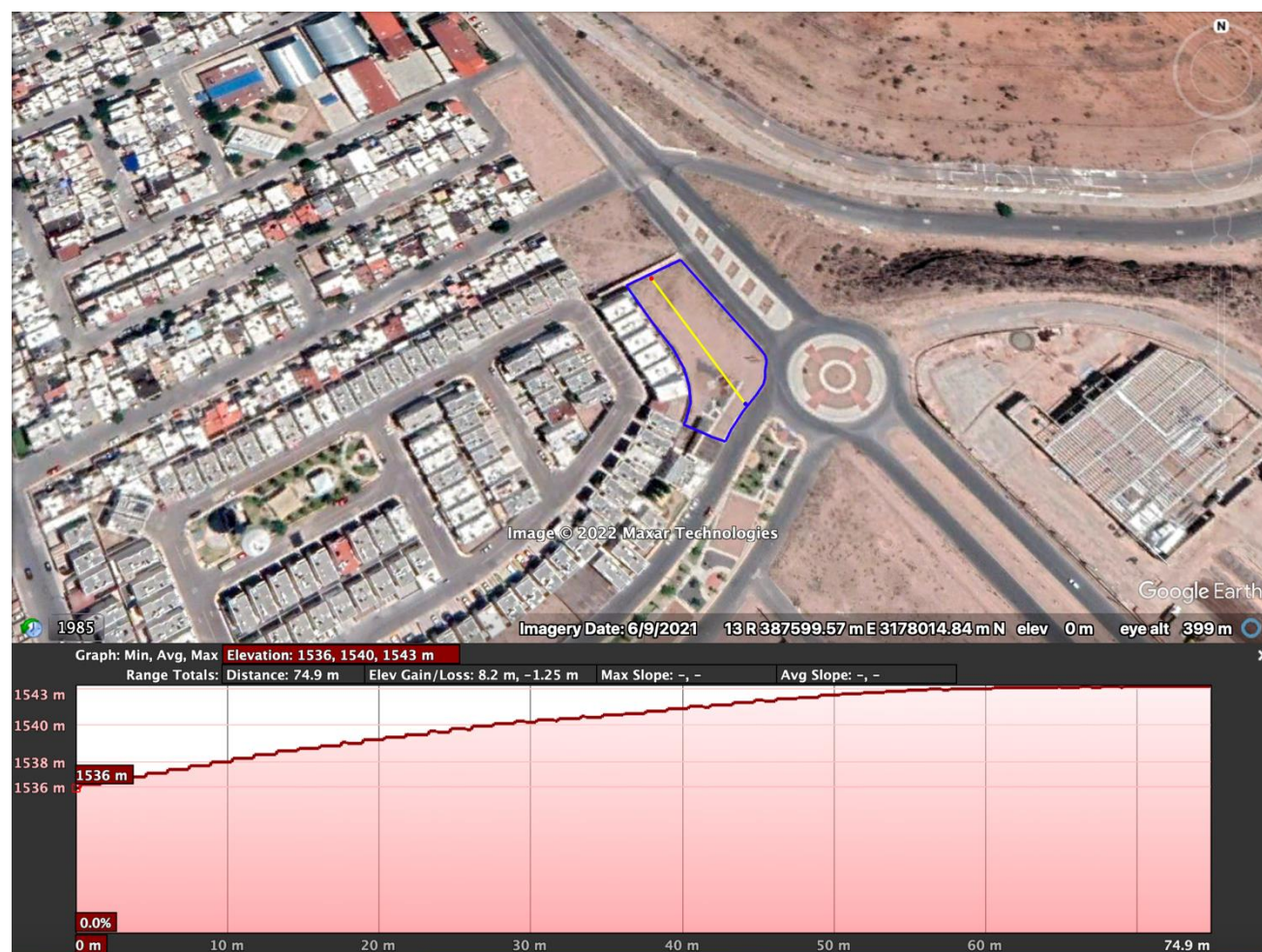
Ilustración 23. Perfil de Elevación transversal. Fuente: Elaboración propia con información de Google Earth, 2022.
