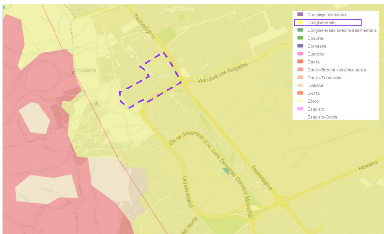
Ilustración 20. Plano de Geología. Fuente: Elaboración propia con información de INEGI, 2020.
